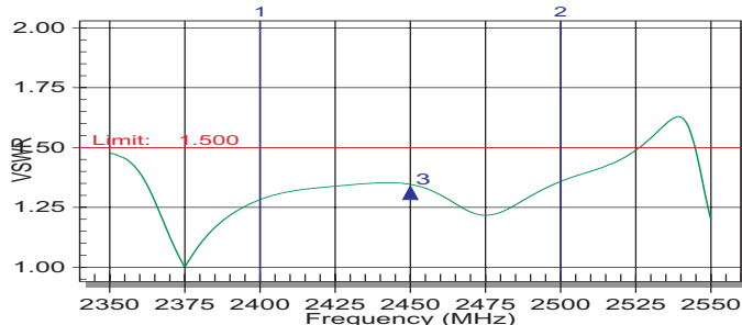
Н Диаграми на излъчване V VSWR Frequency: 2350 MHz - 2550 MHz (Full Cal) MS2412 9/6/2005 4:50:00 PM
