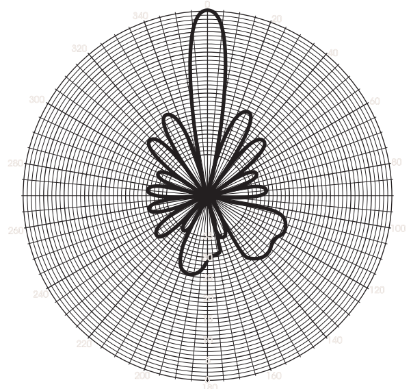
ДИАГРАМА на АНТЕНАТА
